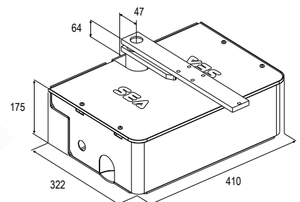
12710400 AP180 Kit for opening up to 180° with chain (max leaf opening 2 m) Ouverture à 180° à chaîne (vantail max 2 m)
